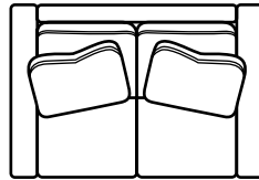
731-019 2-Over-2 Loveseat 57W 39 D 37 H 26 AH 19 SH
